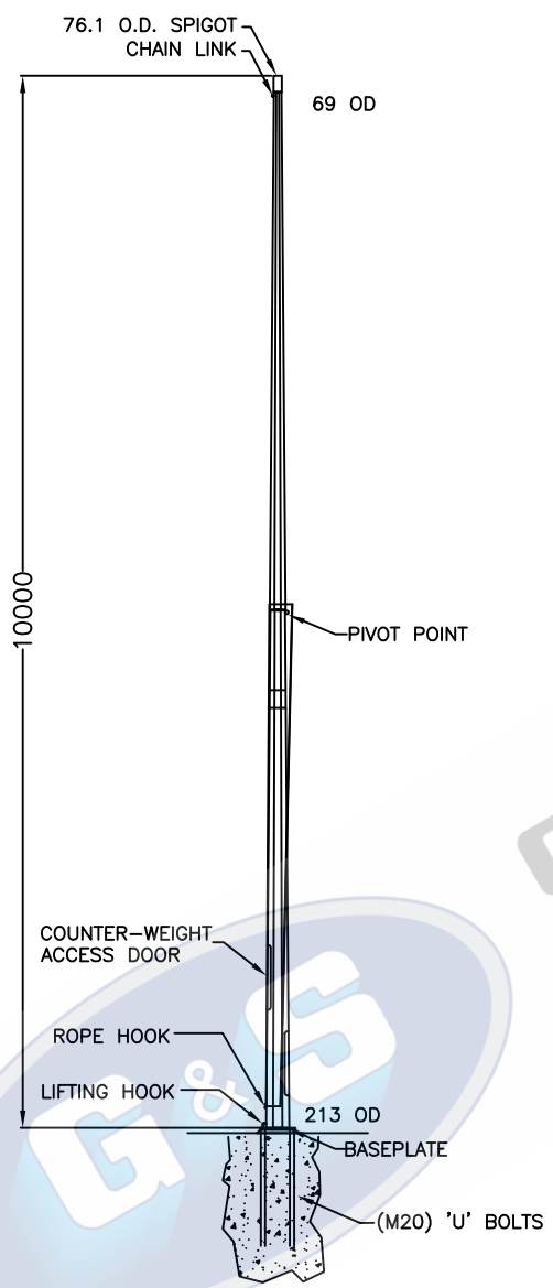
ELEVATION
